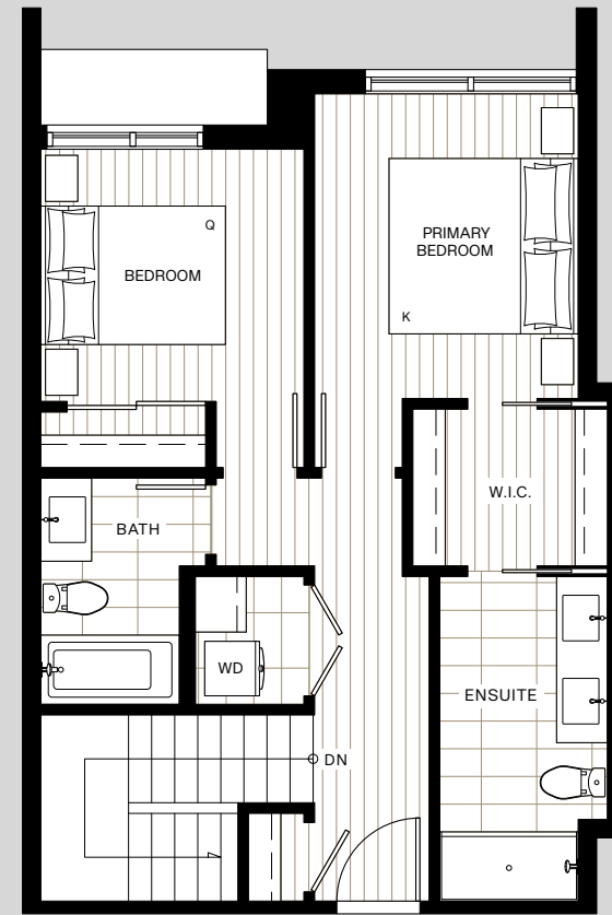
UPPER
